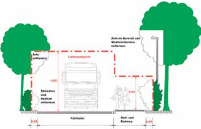
Skizze zum Lichtraumprofil
