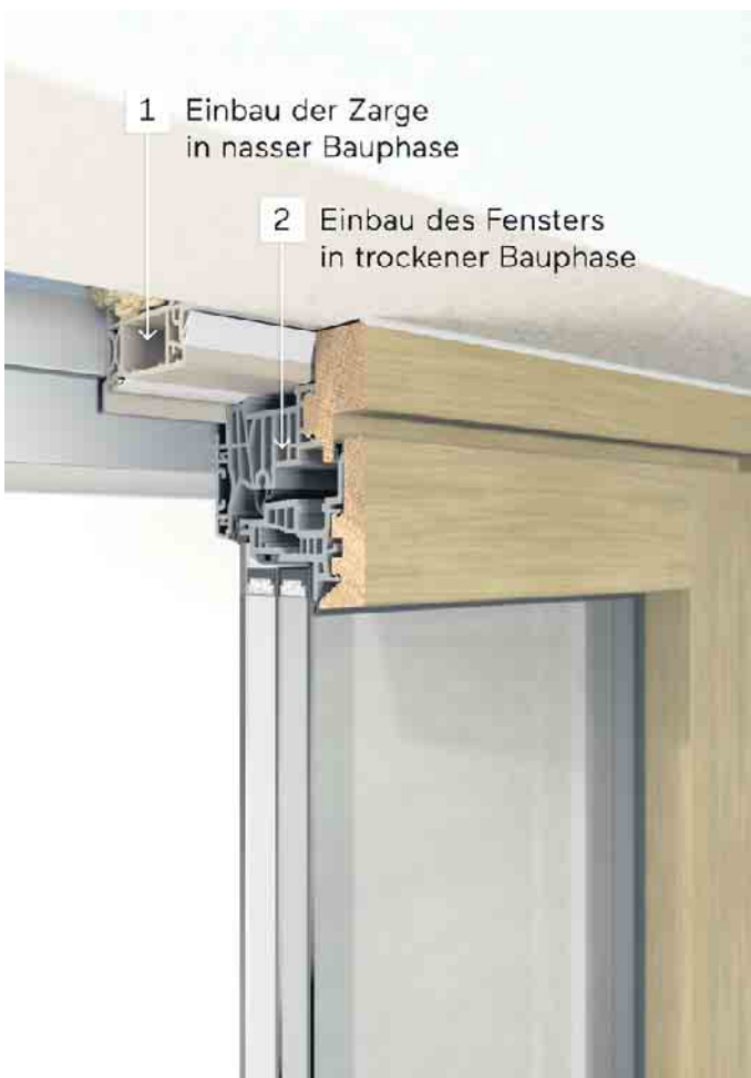
Ein zweistufiger Fenstereinbau mit Einbaurahmen bietet viele Vorteile. Foto: © Finstral
