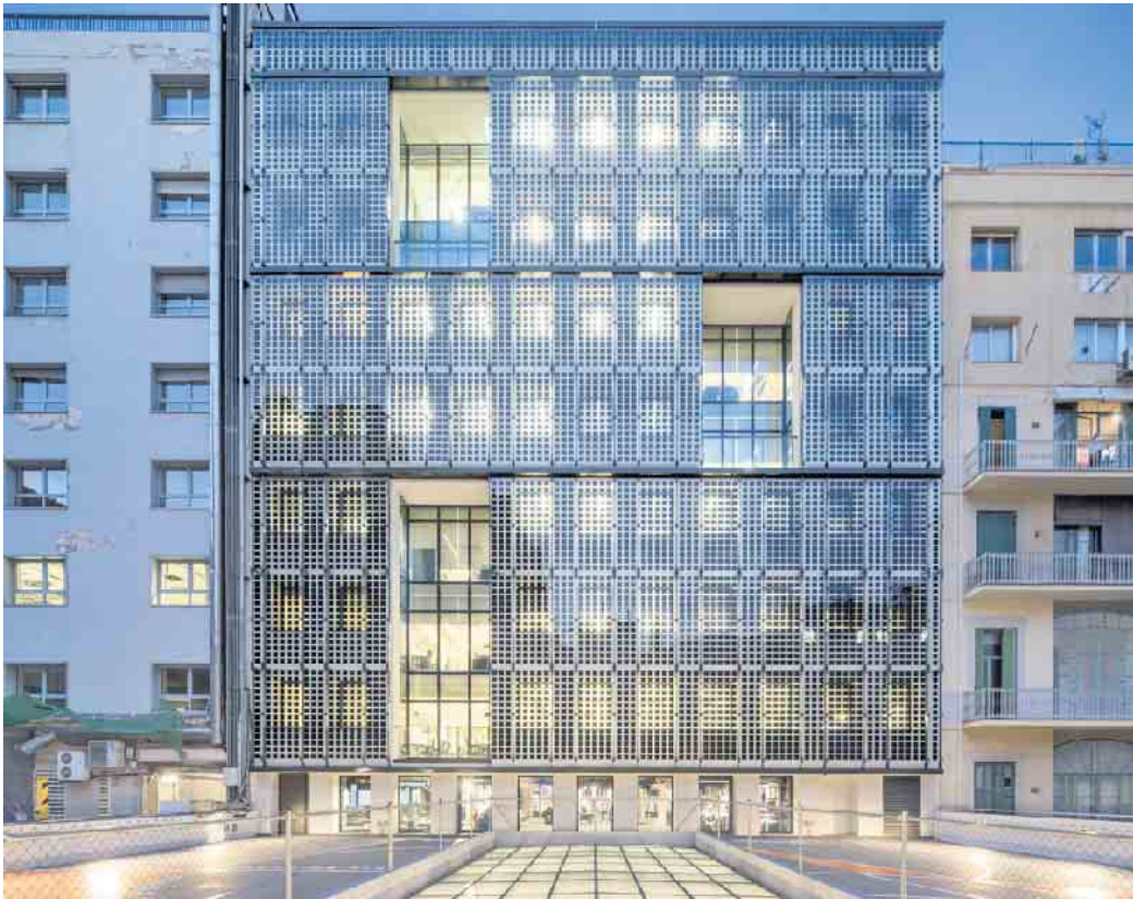
Gut für Klimabilanz und Energieausbeute: Eine vorgehängte BIPV-Lösung an der Fassade einer Gewerbeimmobilie. Copyright: AGC Glass Europe
