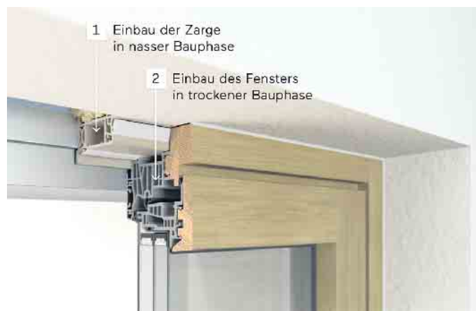
Ein zweistufiger Fenstereinbau mit Einbaurahmen bietet viele Vorteile. Foto: © Finstral
