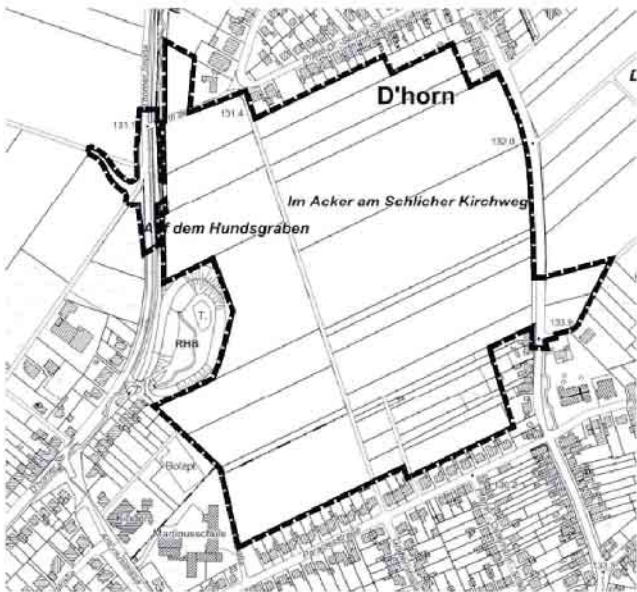
----- Geltungsbereich des Bebauungsplanes C 14
