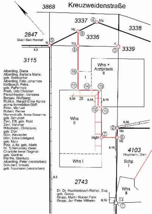
Skizze (unmaßstäblich):
