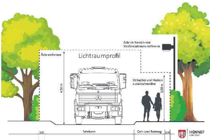
„Lichtraumprofil“ und Pflanzenschnitt: Das sind die Regeln.
