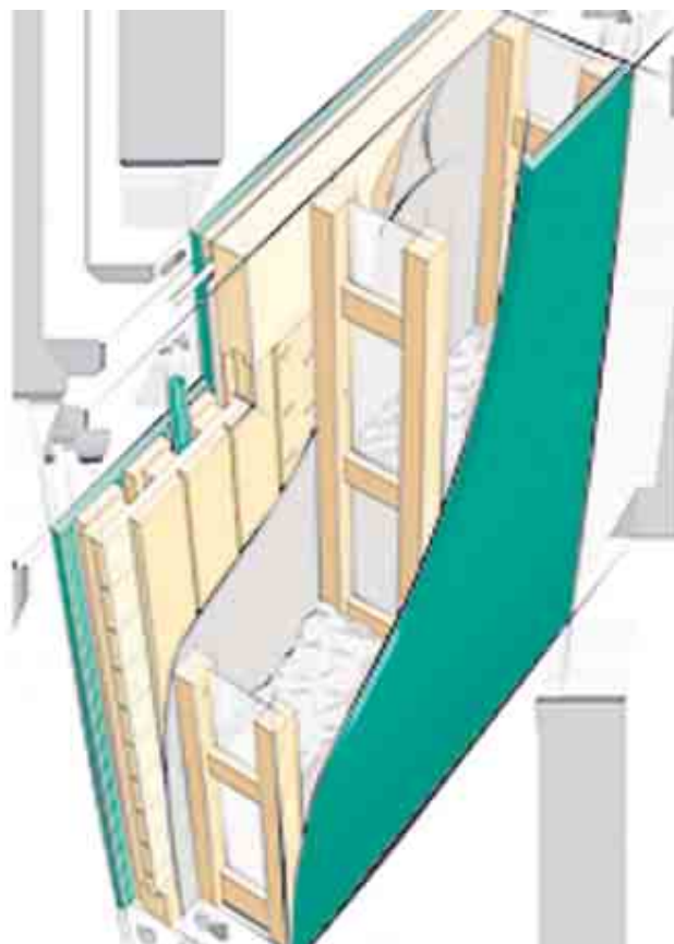
Brettspertholz-Dämmständer; Quelle: www.lignotrend.com
