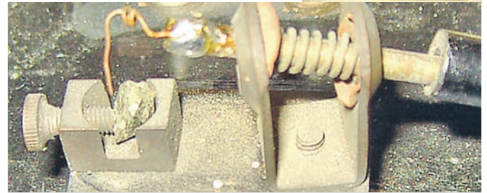
Kristalldetektor (z.B. mit „Teufelsgold“-Kristall zur Gleichrichtung der elektromagnetischen Welle: Man musste so lange probieren, bis man auf dem Kristall eine passende Kontaktstelle gefunden hatte!
